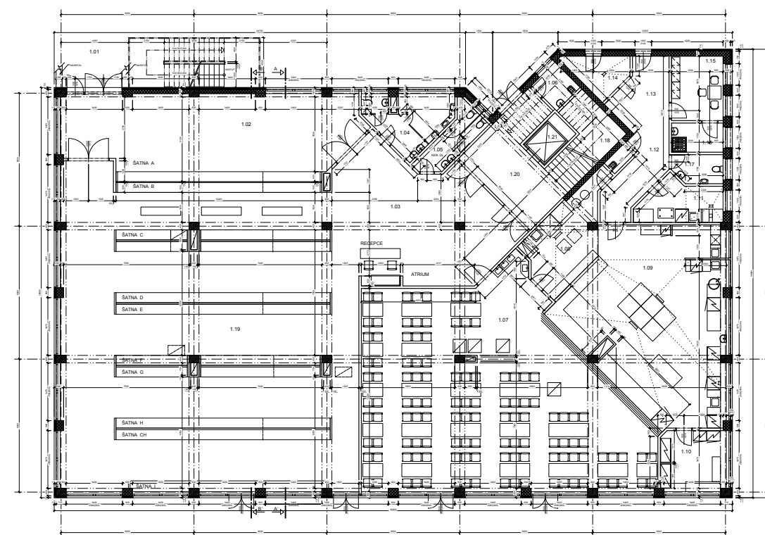
1.NP - PŘÍZEMÍ 1:100
