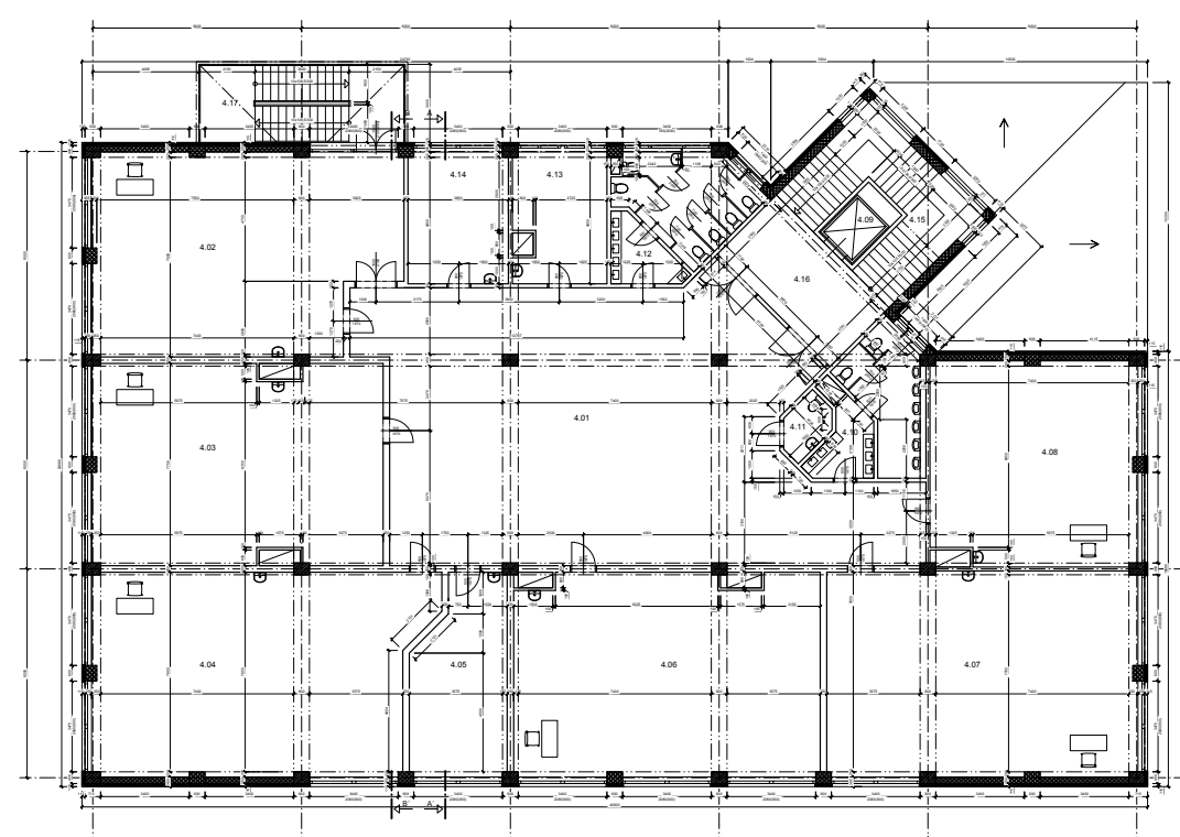
4.NP - 3.PATRO 1:100
