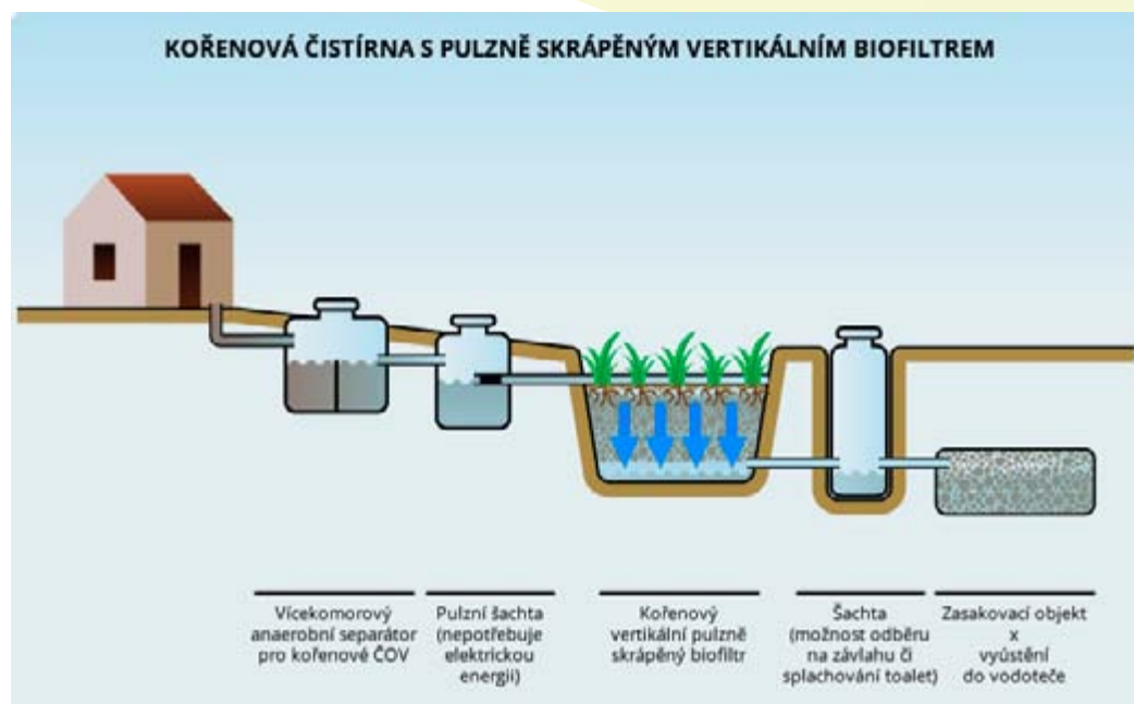
Obr. 1: Schéma kořenové čistírny odpadních vod (zdroj: www.korenovky.cz ).
